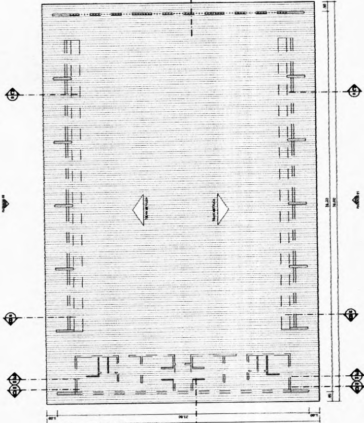
PLANTA DE COBERTURA ESCALA 1:125
